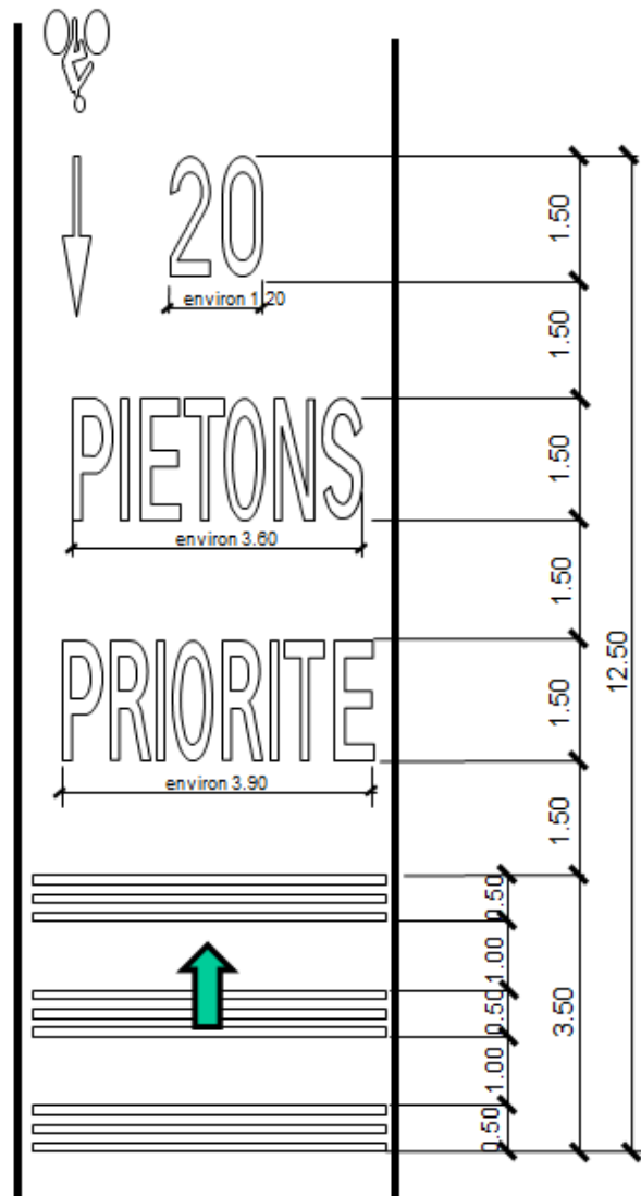
Exemple de marquage sur une chaussée de 4,00m environ
