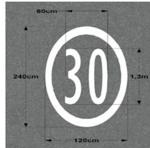
Marquage rappel zone 30 (optionnel)
