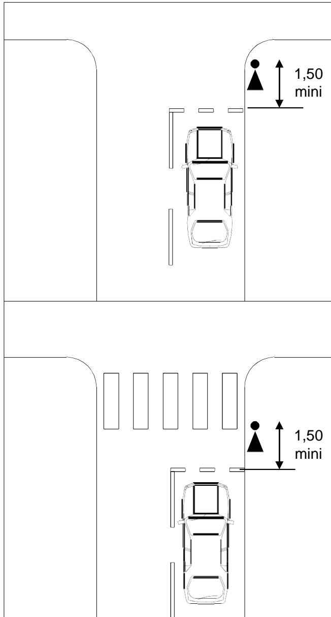
Implantations ligne obligatoire
