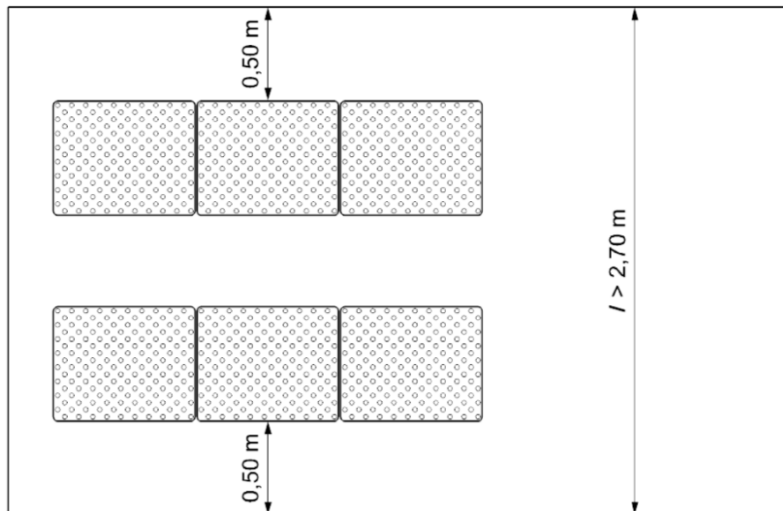
Figure 10 — Implantation sur îlot-refuge de plus de 2,70 m — Bandes de largeur standard
