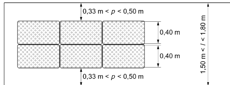
Figure 13 — Implantation sur îlot-refuge de 1,50 m à 1,80 m — Deux bandes de largeur réduite
