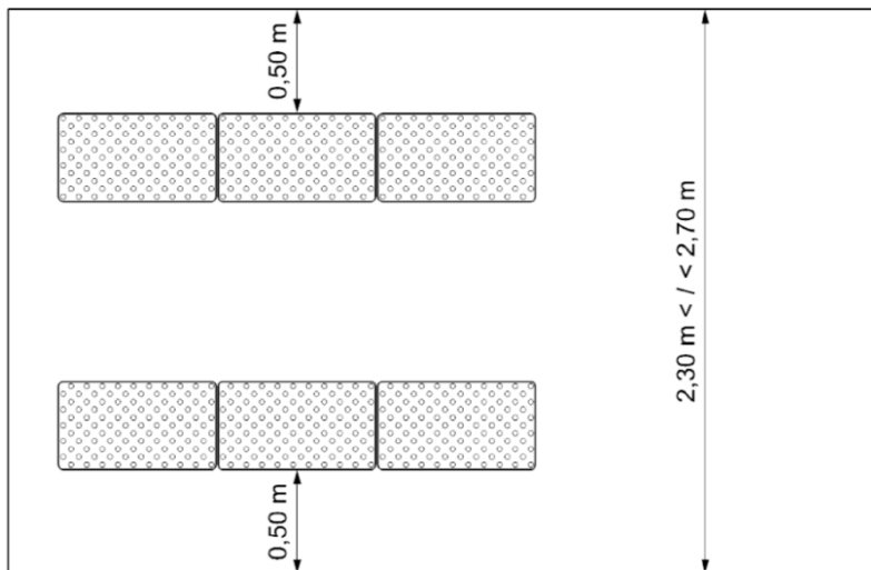
Figure 11 — Implantation sur îlot-refuge de 2,30 m à 2,70 m — Bandes de largeur réduite
