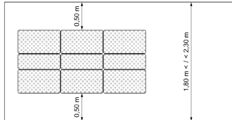
Figure 12 — Implantation sur îlot-refuge de 1,80 m à 2,30 m — Espace comblé entre deux bandes de largeur réduite
