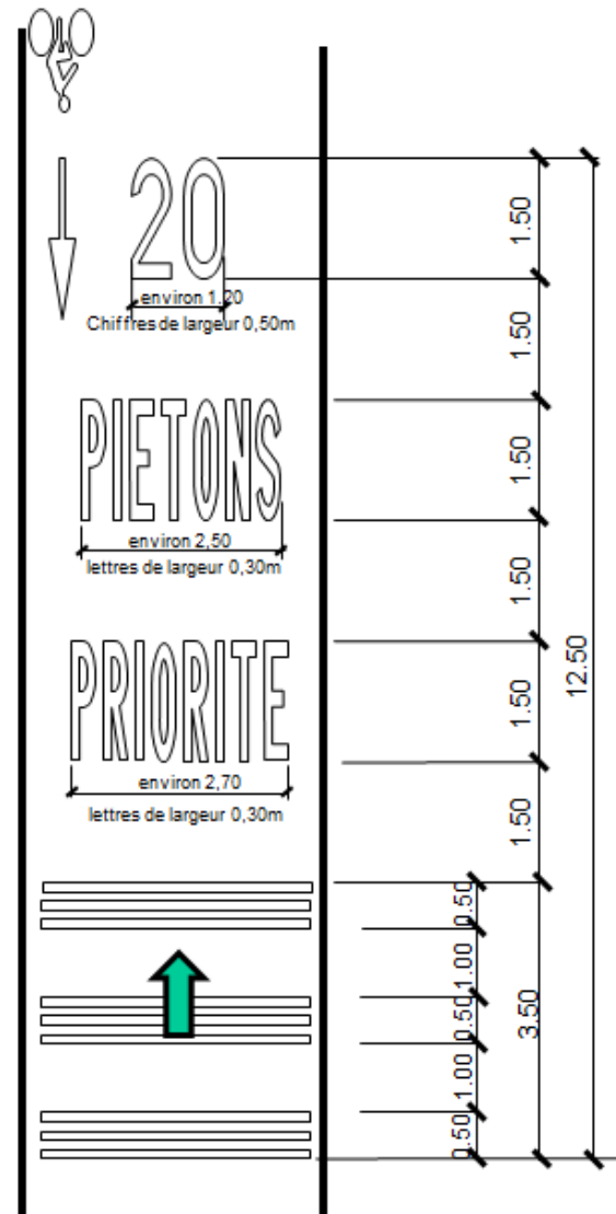
Exemple de marquage sur une chaussée de 3,50m environ
